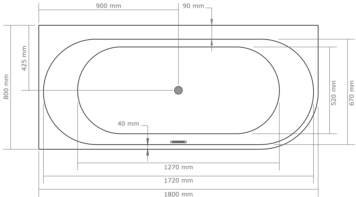
Vue supérieure
